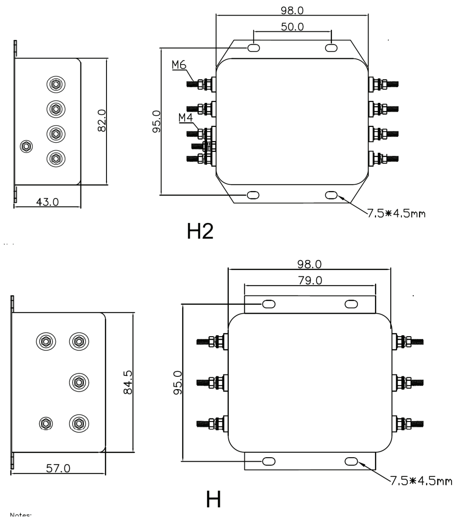
外形尺寸 Outline Dimensions(mm)
